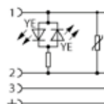
11.024-K, 3-pin + PE
